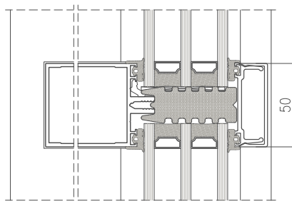
PRZEKRÓJ PRZEZ RYGIEL FA50N HI
