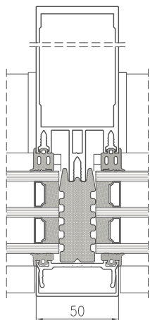
PRZEKRÓJ PRZEZ SŁUP FA50N HI
